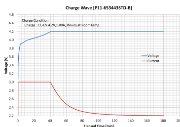
充電波形
