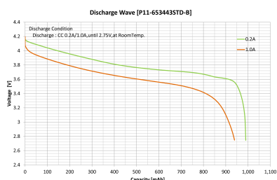
放電波形
